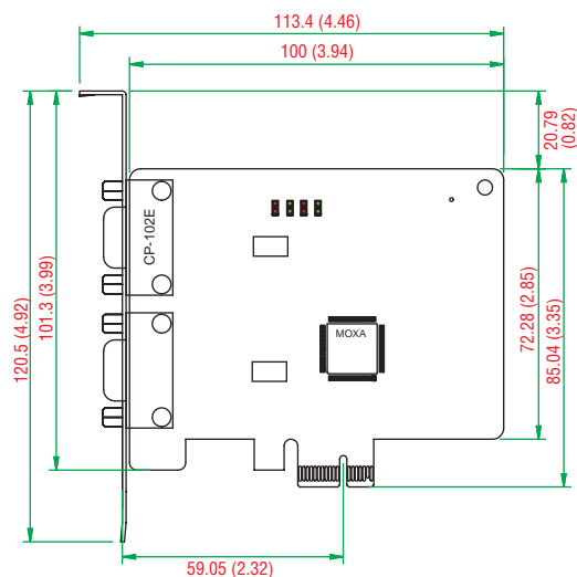
CP-102E
