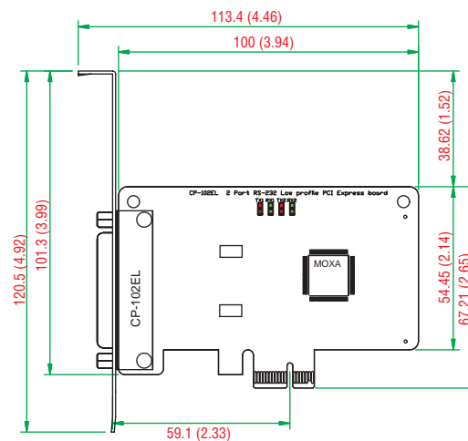
CP-102EL
