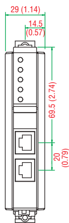
NPort IA5150 NPort IA5150I NPort IA5250 NPort IA5250I
