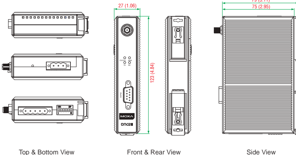
OnCell G2151I
